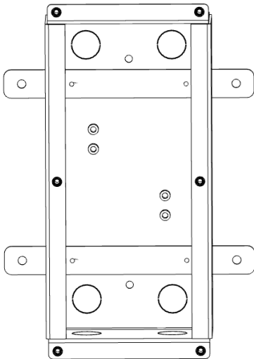
Puszka podtynkowa
